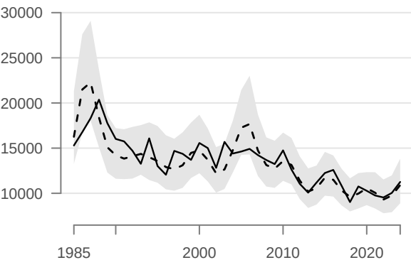
Estimation error
